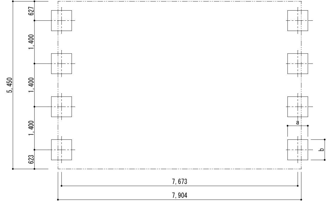
■ 基礎配置図
